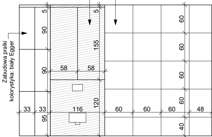
WIDOK E-E
