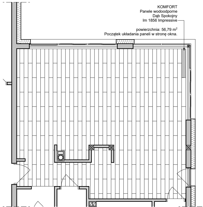
UKŁAD PODŁOGI
