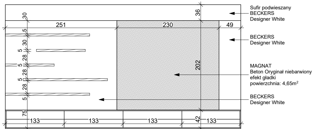
WIDOK G-G
