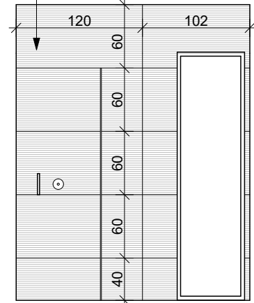
WIDOK F-F
