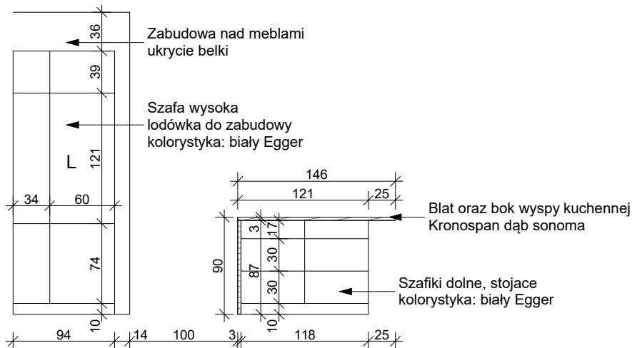
WIDOK B-B
