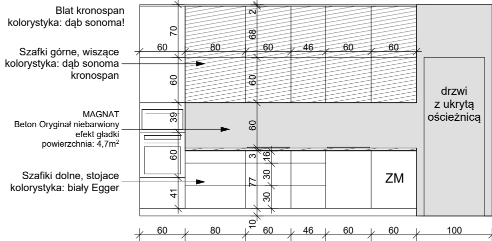
WIDOK A-A
