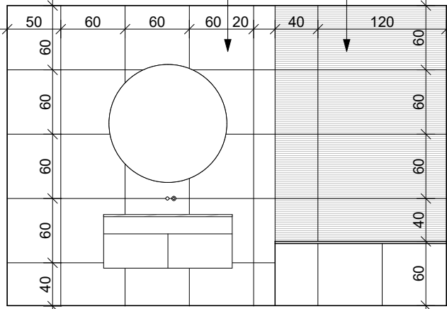
WIDOK C-C
