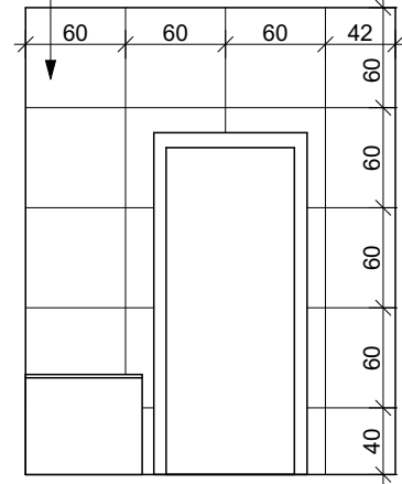
WIDOK D-D
